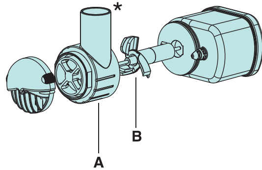
BOMBA CENTRÍFUGA 600
