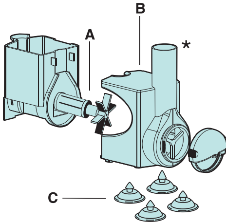
BOMBA CENTRÍFUGA 1000/1200
